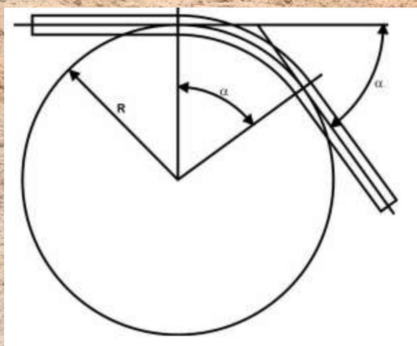
Rys.1 Gięcie rur PE
